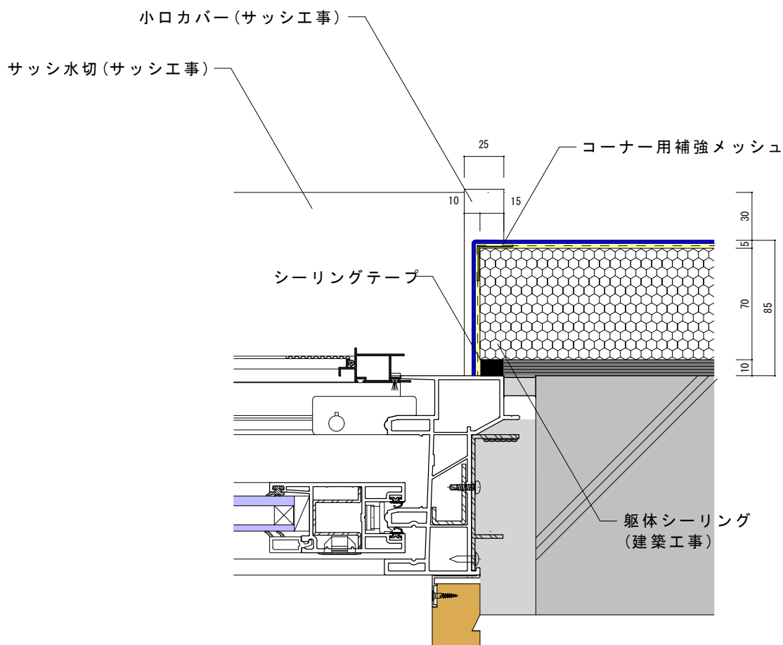
サッシ取合平面図
